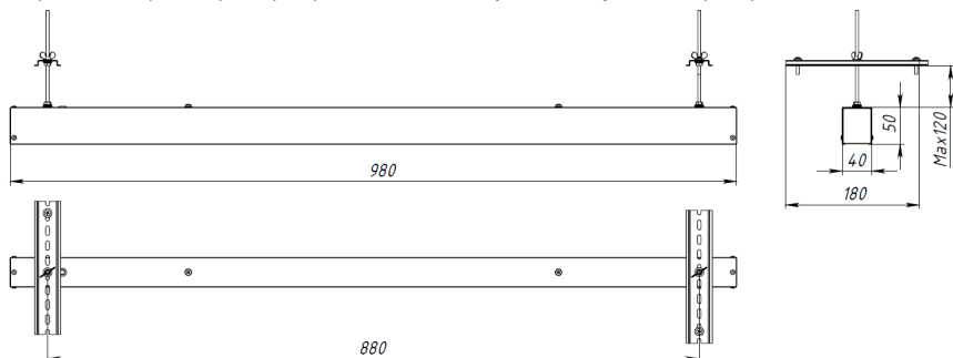
Рисунок 3 - Габаритные размеры при комплектации с креплением уголок на примере Line 980мм.
